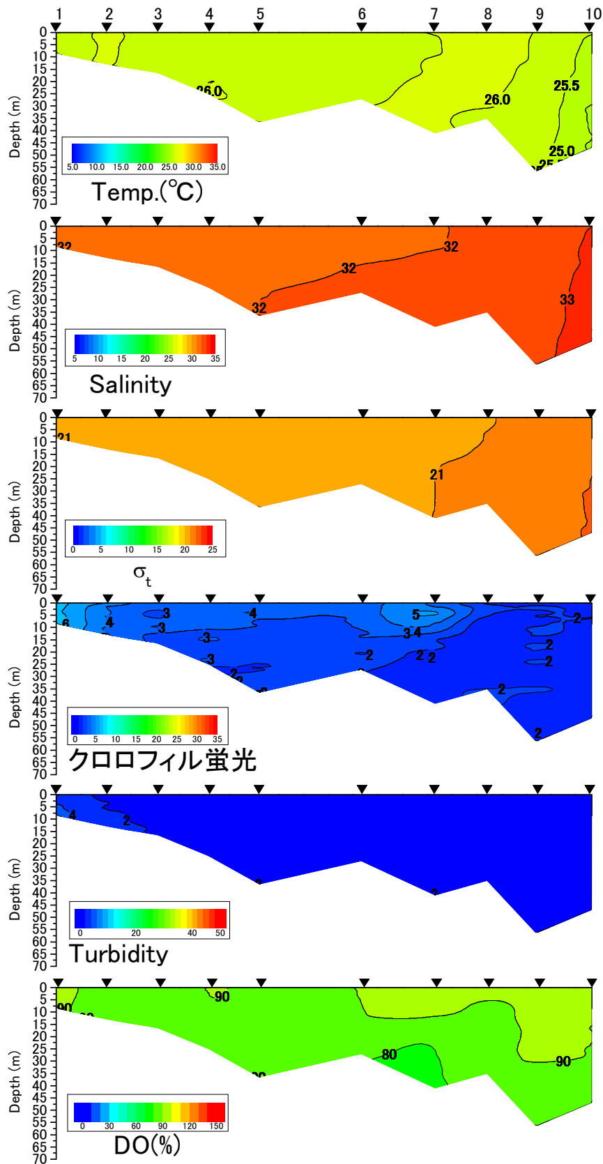
有明海中央ラインの水温(°C)、塩分、密度( \sigma_t )、クロロフィル蛍光強度、濁度、溶存酸素飽和度(DO%)の鉛直面図(国土交通省の調査による) (2016年9月1日)
